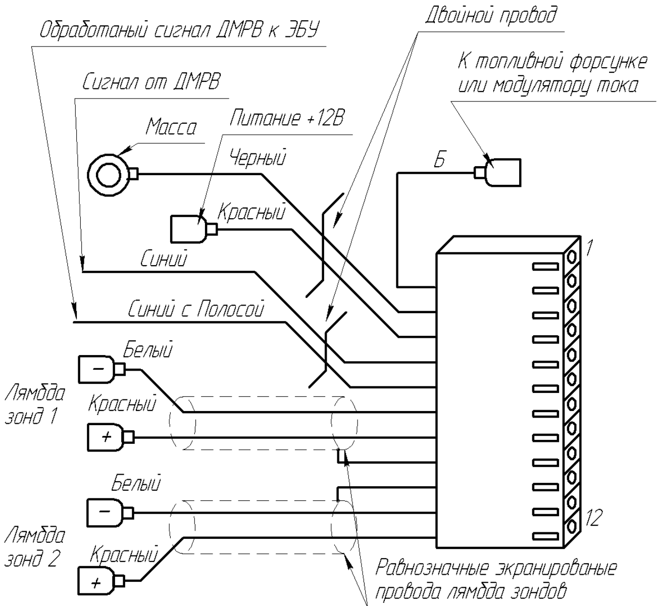
Рисунок 3.3. схема подключения оптимизатора
