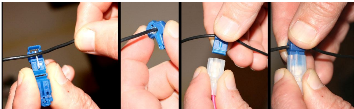
Рисунок 3.2. Методика подключения проводов при помощи быстрых соединителей.
